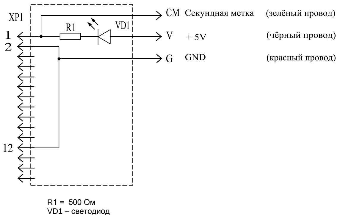
Рисунок 9 – Монтажная схема измерительного разъема
