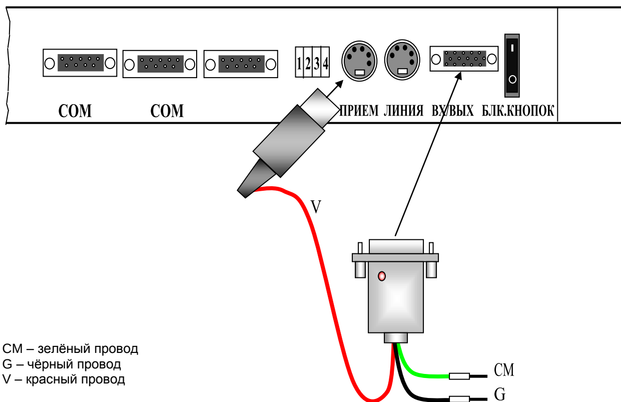
Рисунок 10 – Подключение измерительного разъема к ИБЧ-1/С, ИБЧ-1/СП, ИБЧ-1/СВ, ИБЧ-1/СВП, ИБЧ-1/СЧ, ИБЧ-1/С/ТВ, ИБЧ-1/СП/ТВ, ИБЧ-1/СВ/ТВ, ИБЧ-1/СВП/ТВ
