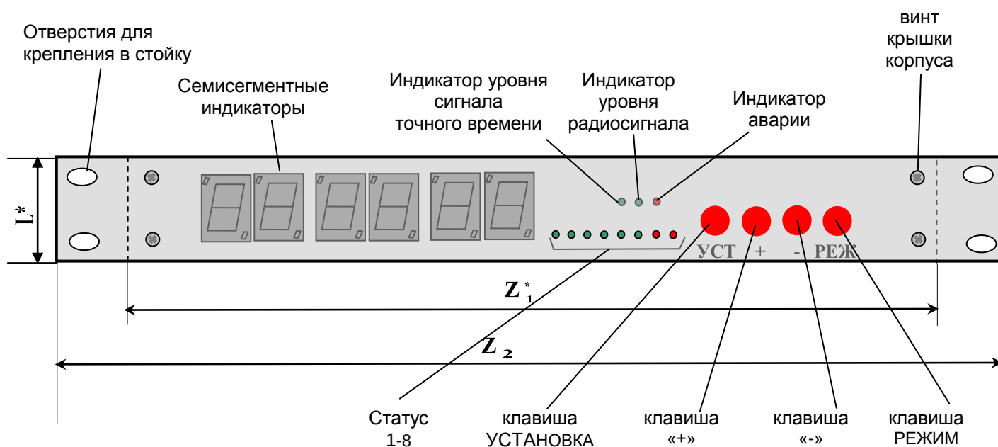
Рисунок 3 – Органы управления и подсоединения ИБЧ-1/С. Вид спереди
